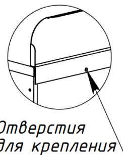
Схема установки заднего борта
